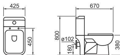
UC11011P Monoblok baltik - komplet Priključak vode sa donje leve strane
