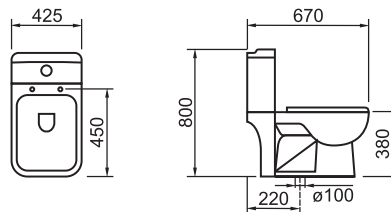
UC11011S Monoblok simplon - komplet Priključak vode sa donje leve strane
