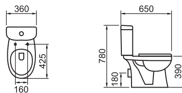
055A-P Monoblok baltik - komplet Priključak vode sa donje leve strane
