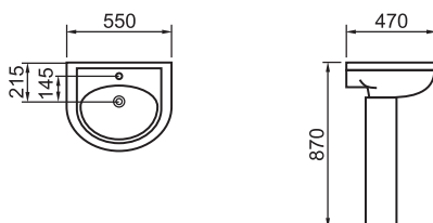
013B Lavabo sa stubom (širina 55 cm)
