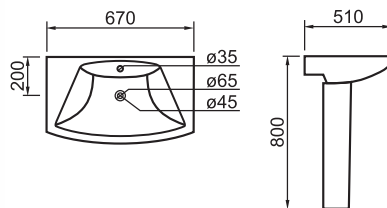
UC915 Lavabo sa stubom (širina 67 cm)
